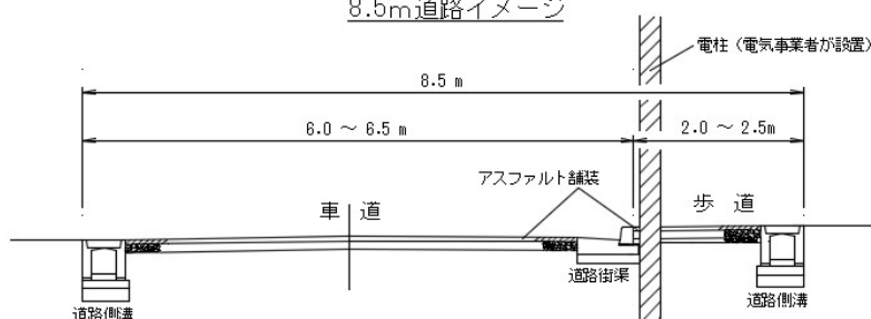
8.5m道路イメージ
