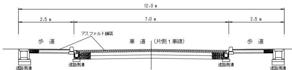
都市計画道路 甲子園段上線 整備イメージ
