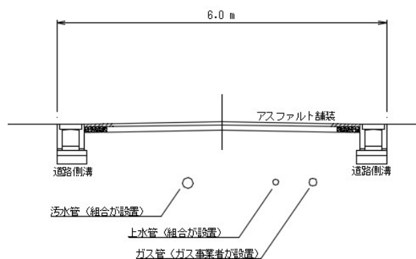
6.0m道路イメージ
